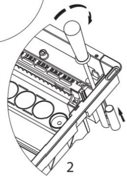
Halter für sichere Montage bei der Montage bei Hohlraumwänden
