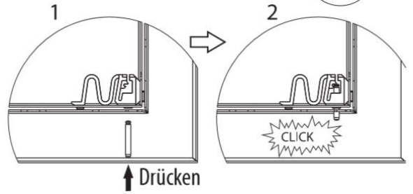
Türaufhängung rechts oder links
